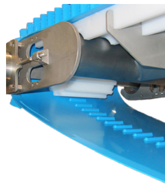
BANDA TRANSPORTOARE
